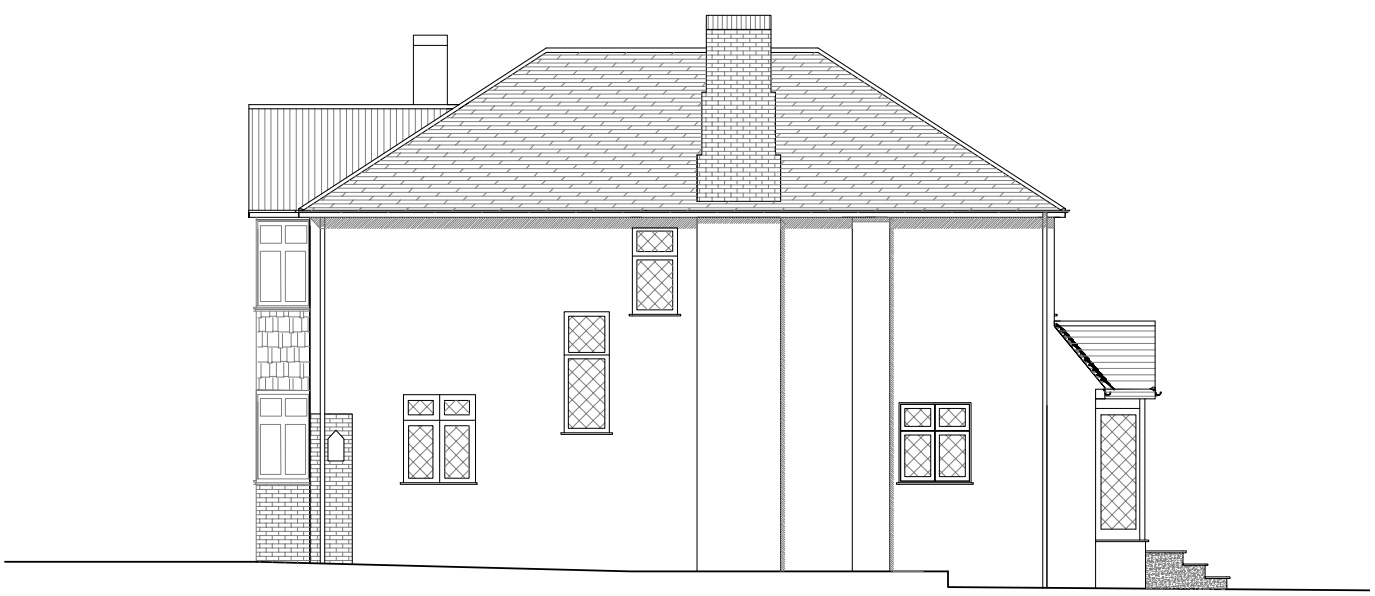
Flank Elevation
