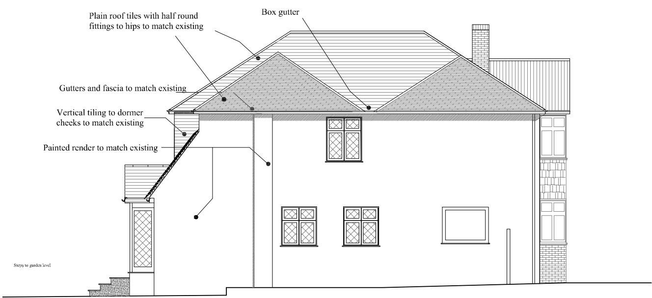
Flank Elevation
